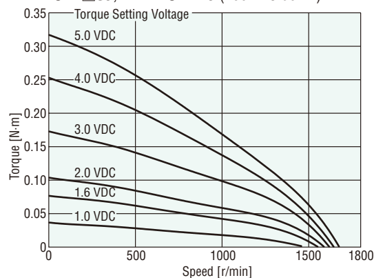
TM410A-□SJ, TM410A-AJ (100 VAC 60 Hz)
