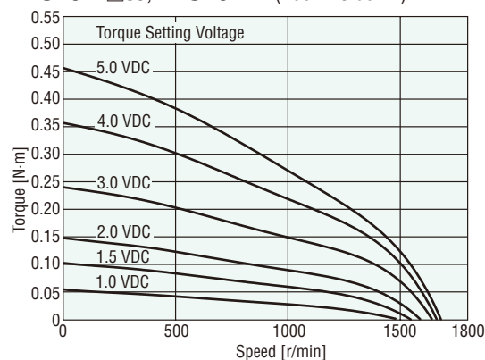
TM520A-□SJ, TM520A-A (100 VAC 60 Hz)
